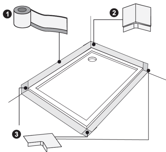
(1) Bande d'étanchéité (2) Angle entrant (3) Angle multifonction
